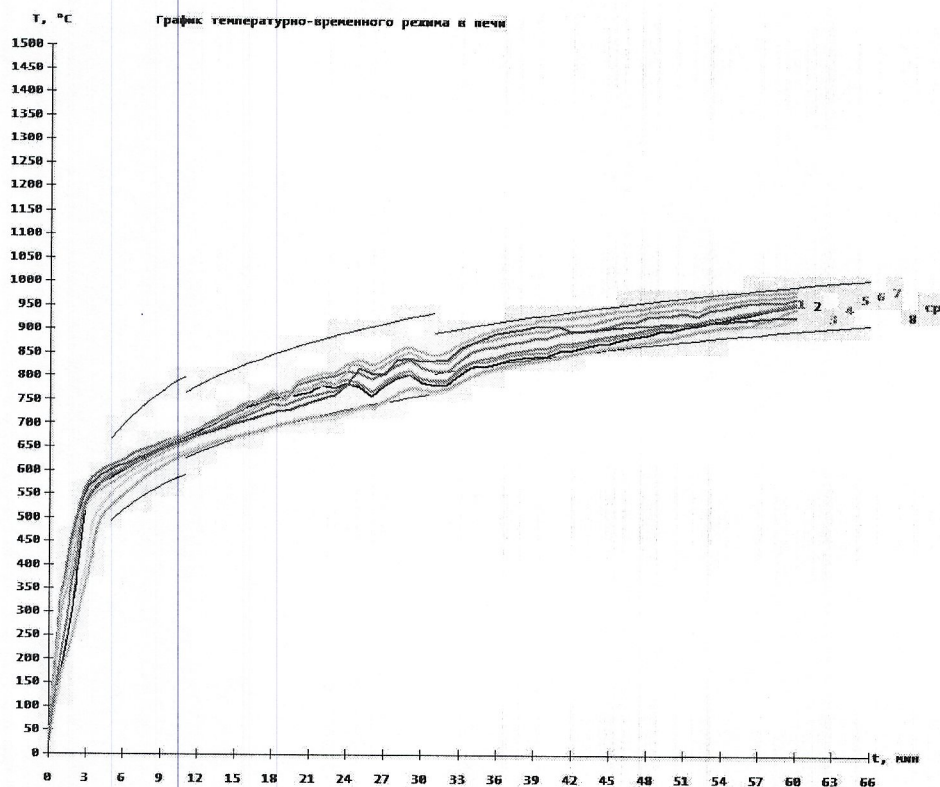
График изменения температурно-временного режима в объеме печи
