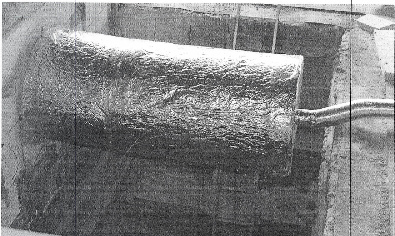
Вид образца после испытания
